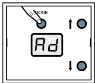
Solange die MODE-Taste kurz gedrückt wird, wird „Ad“ auf dem Display angezeigt.
